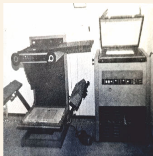
Reprokamera und Kopierrahmen zum Herstellen von Druckplatten
